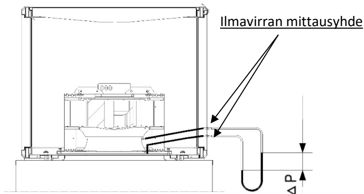
Ilmavirranmittaus ECO 30 – 40
