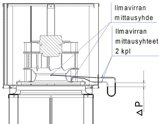
Ilmavirranmittaus ECO 03 – 20
