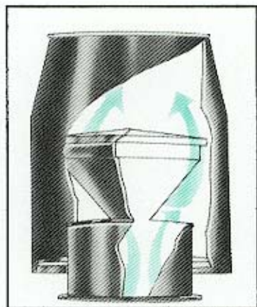
PERIAATEPIIRROS
