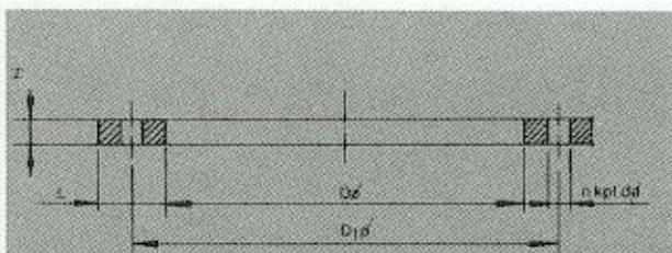
Liitântälaippa
