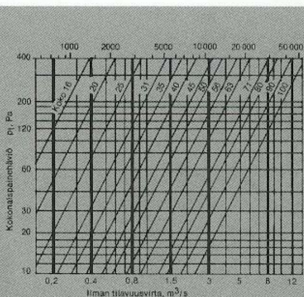
Painehäviö
